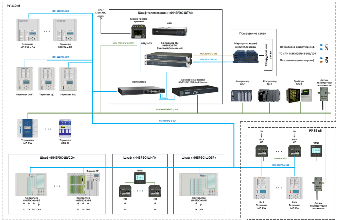
Структурная схема ПТК ИНБРЭС для ССПИ ПС 35-110 кВ
