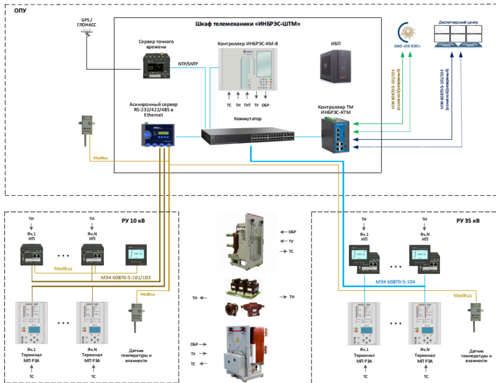
Структурная схема ПТК ИНБРЭС для ССПИ/ТМ ПС 6-35 кВ
